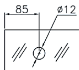
NOB-861 DOOR KNOB
