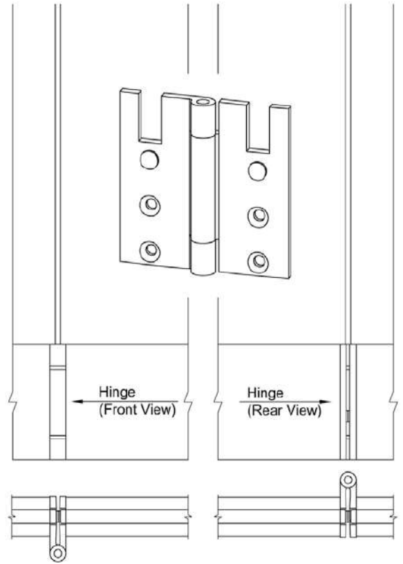
Door Rail c/w Hinge
