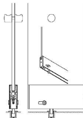
Bottom Rail c/w Lockset
