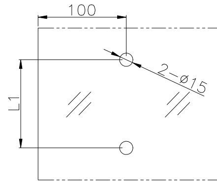
GLASS PREPARATION (N.T.S)
